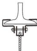
工字吊架 (訂製品)
