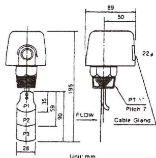
DIMENSION (流量開關)
